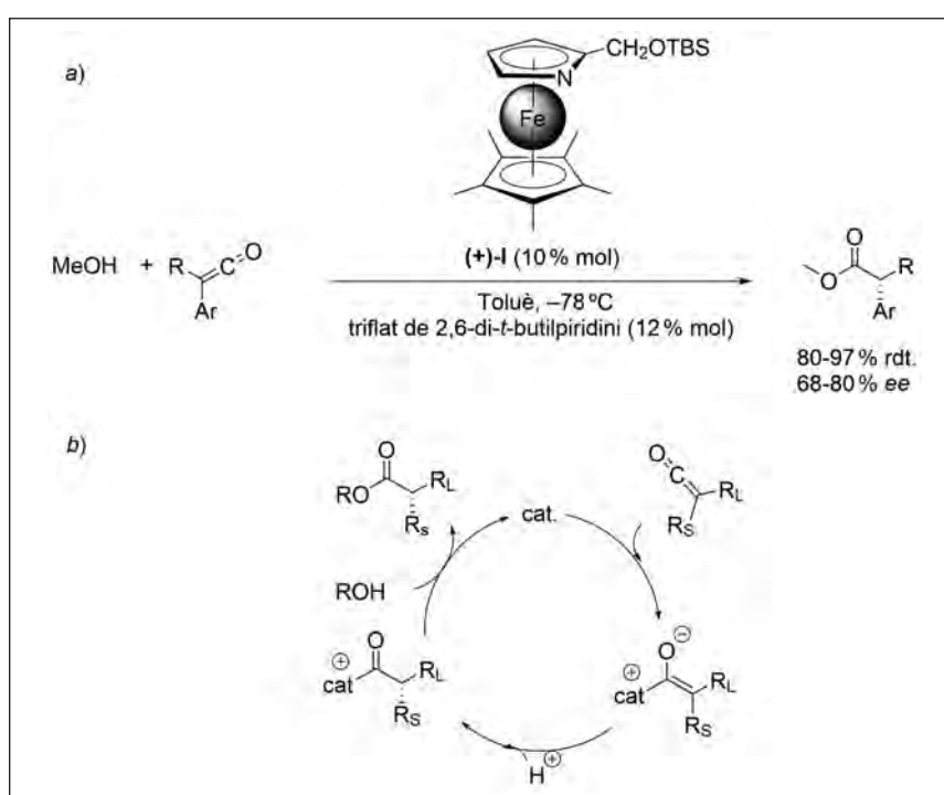
FIGURA 2. Síntesi asimètrica d'èsters catalitzada per l'esfera de coordinació d'un ferrocè quiral. Elaboració pròpia.
